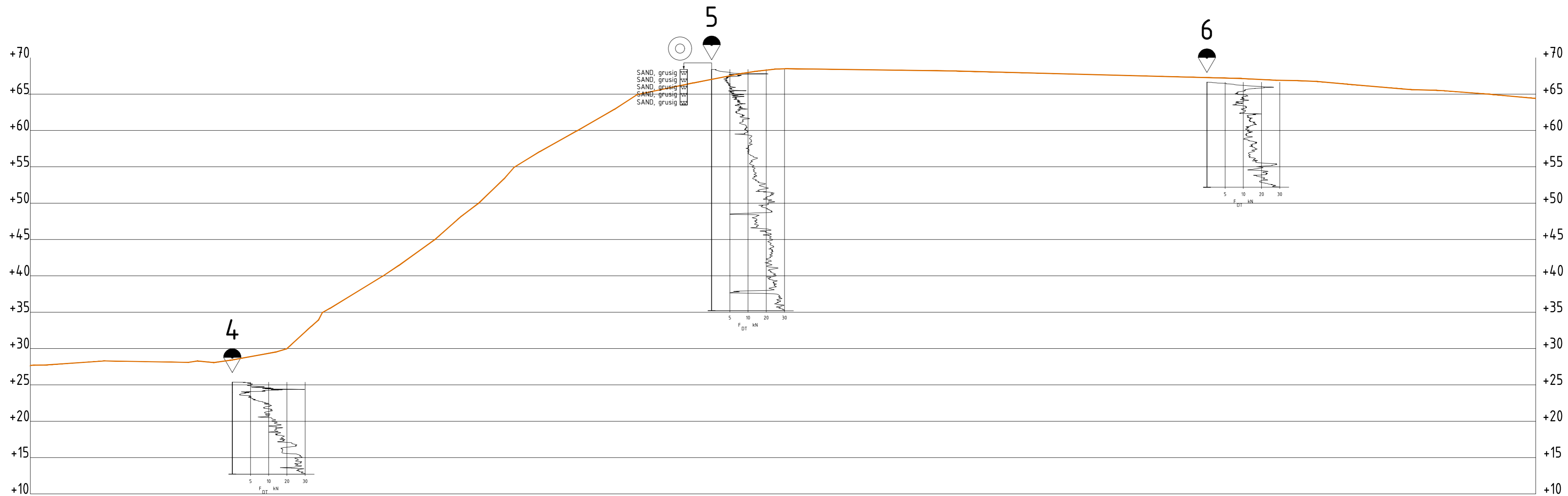
Profil B-B
